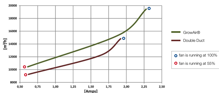
Fan efficiency
